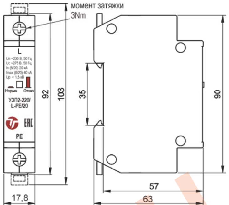
Рис.1 Габаритные размеры
